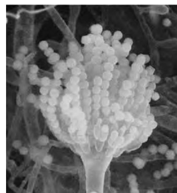
Aspergillus 属糸状菌の分生子形成器官
